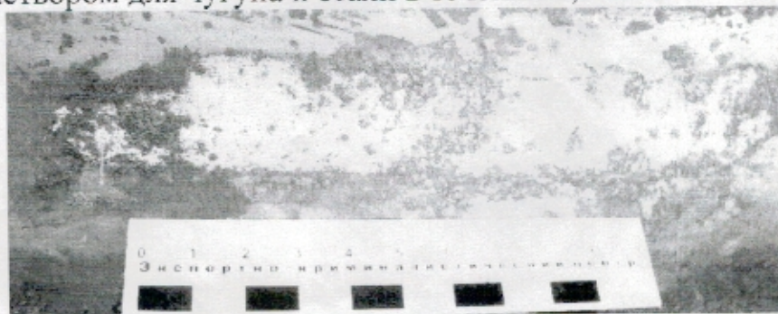
№ 4 Общий вид поля маркировки шасси (VIN), после химического травления.
